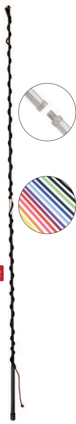
Longierpeitsche , Nylonfaden übersponnen, mit Metallwirbel, PVC-Griff, mit Nylon-Longierschlag, teilbare Peitsche, mit Schraubverschluss Lunging whip , with pvc-grip and swivel, woven nylon cover, two-piece lunging whip, screwable Farben: verschiedene aktuelle Farben/assorted colours 55950 180 cm 55960 200 cm
